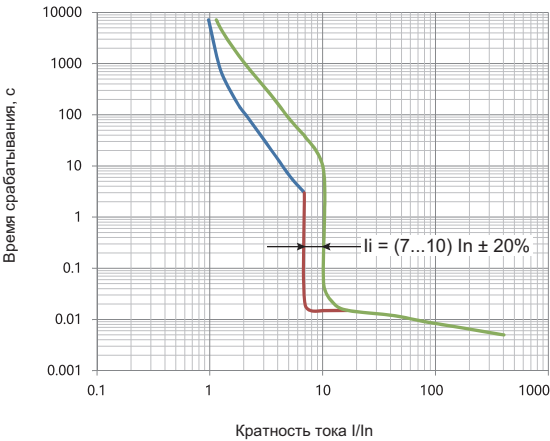
Времятоковая характеристика
