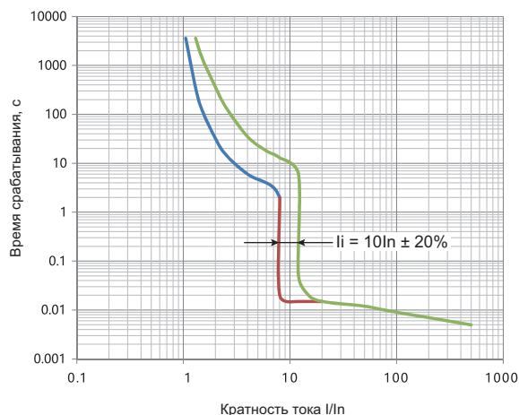
Времятоковая характеристика
