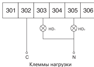
800A-3150A/4 полюса (стандартный тип)
