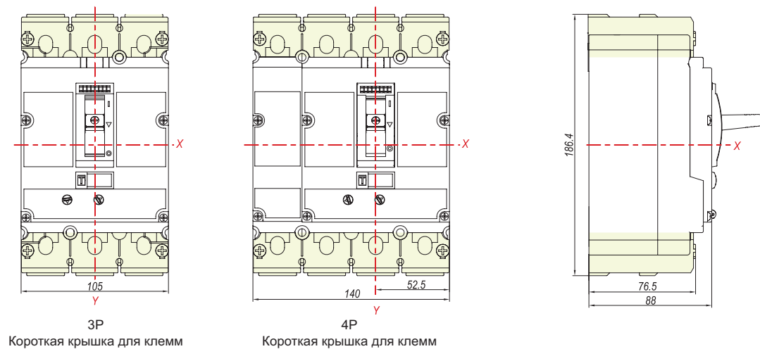
Короткая крышка для клемм
