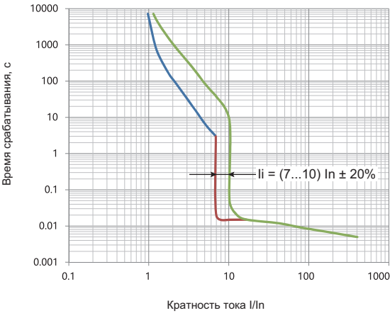
Времятоковая характеристика
