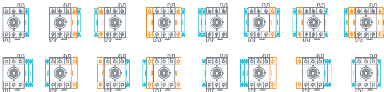
Схема установки дополнительного полюса
