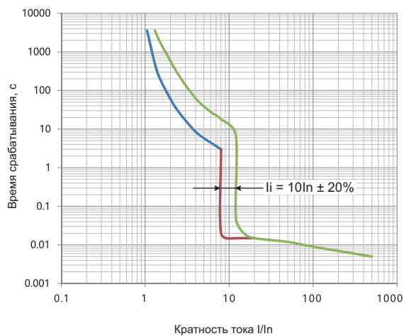
Времятоковая характеристика
